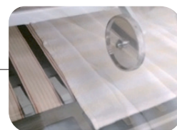
Bypass arrière Sortie à table arrière
