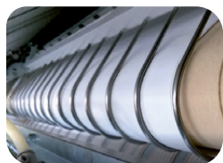
Bypass mécanique 1er pli longitudinal
