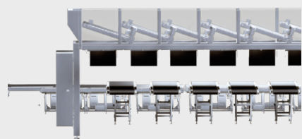
Convoyeurs de pesage + Système de chargement aérien
